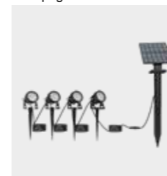
24000/N-C Kit 4 proiettori LED a picchetto in alluminio con pannello fotovoltaico
